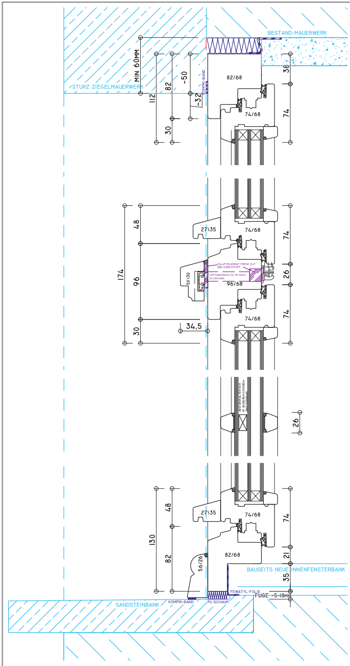
Abb. LÖFFELFENSTER
